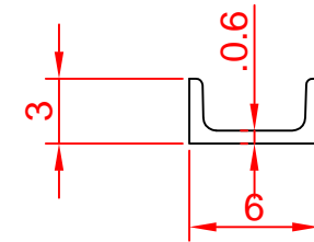
مقطع ناودانی سنگین شماره 6
